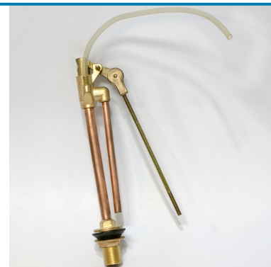
VALVULA ALIMENTADORA P/WC BRONCE
