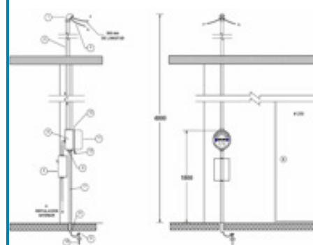
ACOMETIDA COMPLETA P/MEDIDOR
